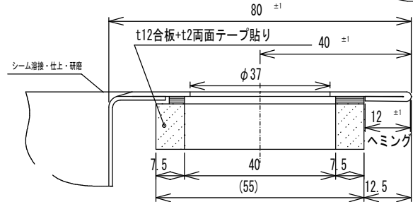
A-A'断面 S=1/1
