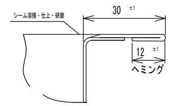
B-B' 断面 S=1/1
