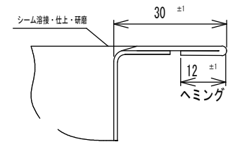
B-B' 断面 S=1/1
