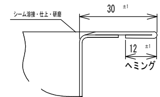
B-B' 断面 S=1/1
