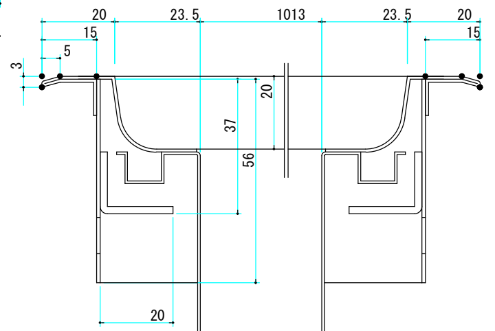
AA断面 (1/1)
