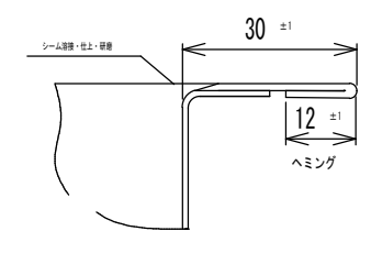
B-B' 断面 S=1/1
