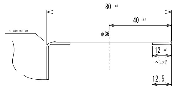
A-A' 断面 S=1/1
