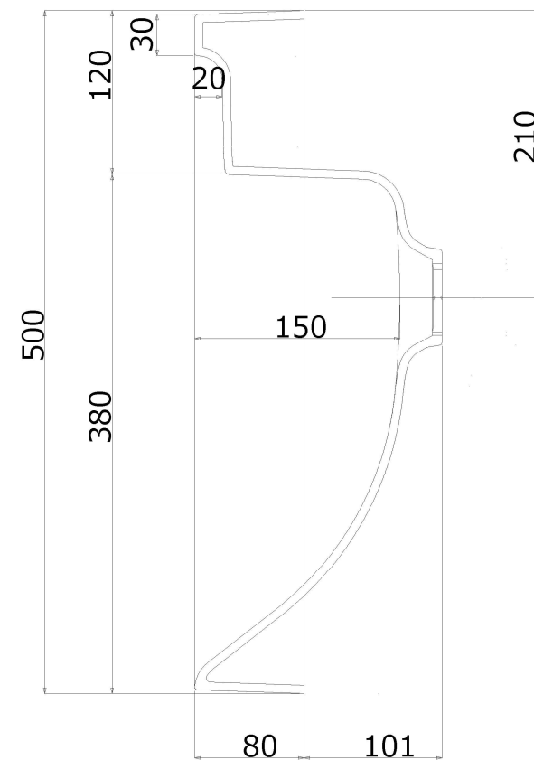
A-A断面図
