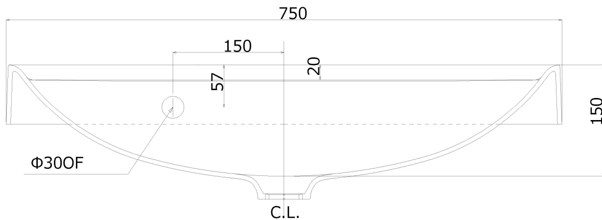
B-B断面図
