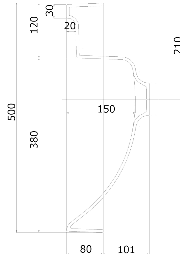
A-A断面図
