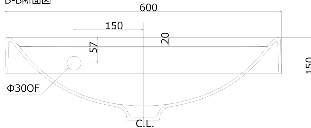
B-B断面図
